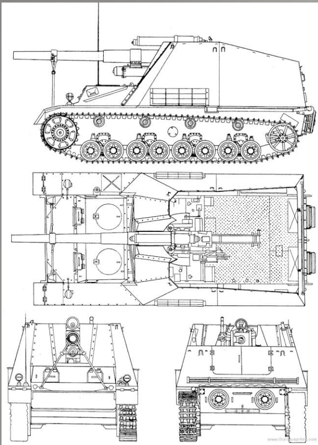
Чертеж САУ «Hummel»
